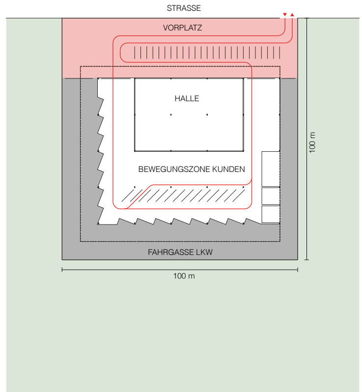
Grundrissvariante Quadrat 100 m x 100 m
