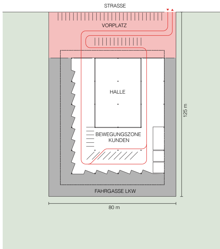
Grundrissvariante Rechteck 80 m x 125 m
