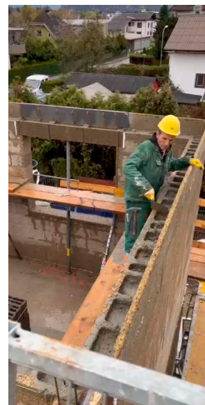
Mauer mit gefüllten Mantelbetonsteinen, Ansicht von oben
